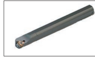
NVRC050-3 D: 0.75" Min. Bore Dia: 0.67" EDP # 66238
